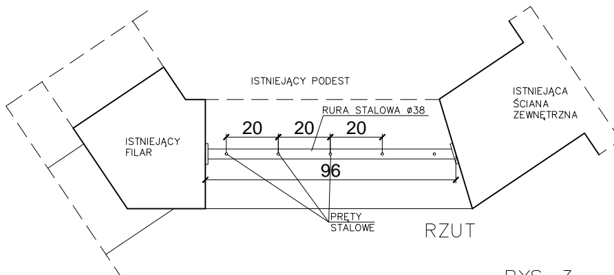
RYS. 3 DETAL BALUSTRADY - 2 SZT.
