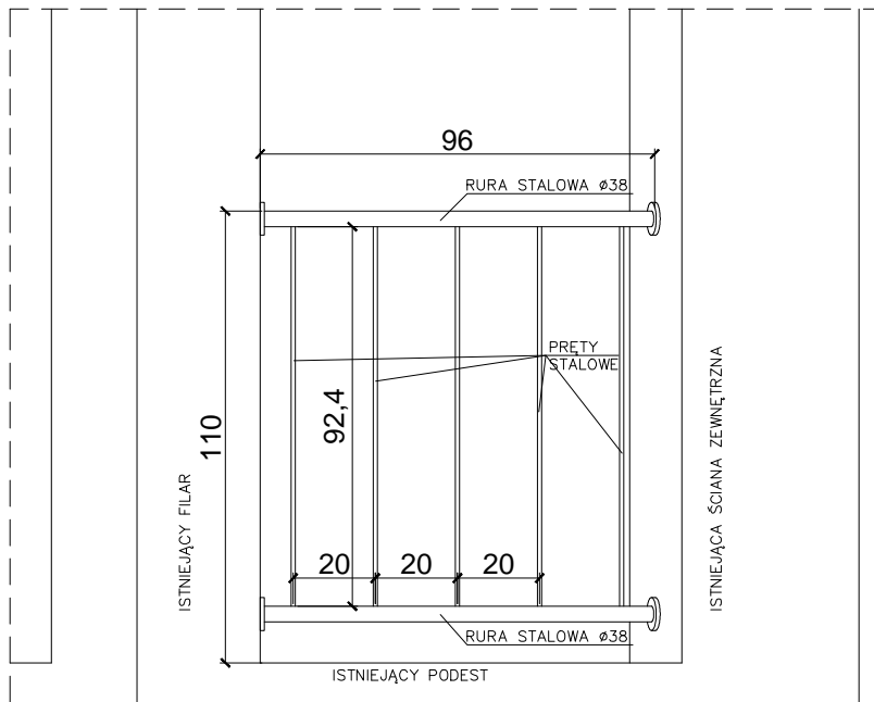
WIDOK
